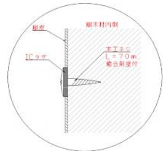
▲ICタグ取付拡大図
