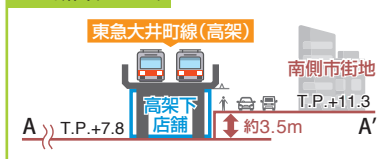
A-A' 断面 (イメージ)
