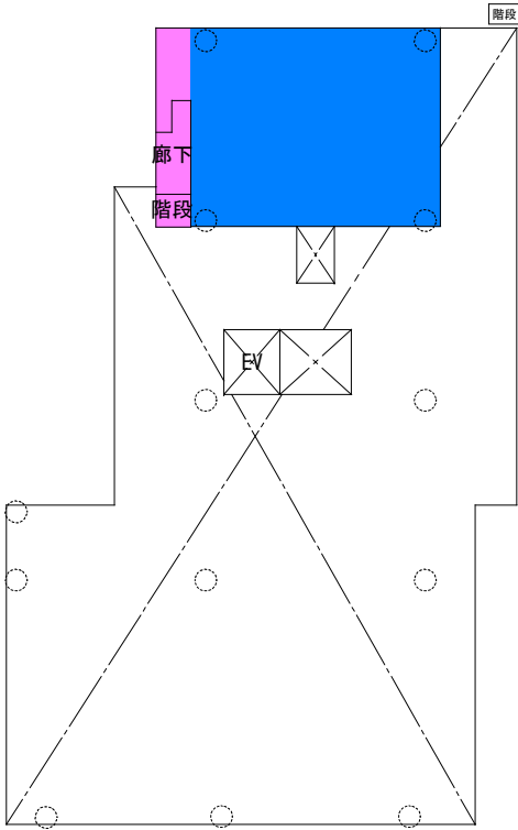
塔屋 1 階平面図
