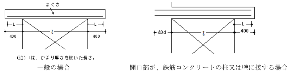
図 8.2.2 鉄筋の定着長さ
