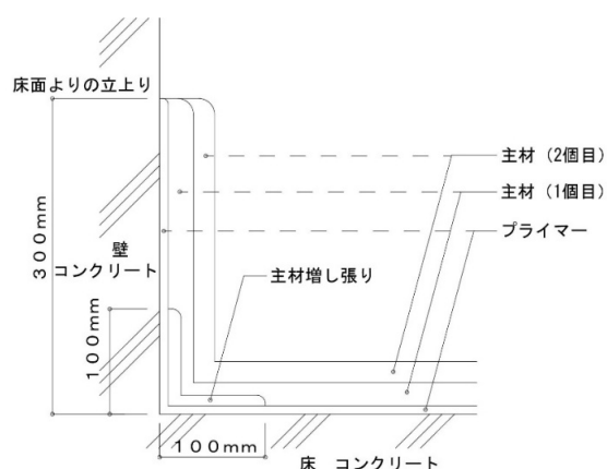
9.5.2 図 主材の施工範囲
