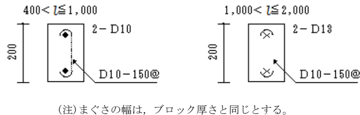
図 8.2.3 まぐさの配筋
