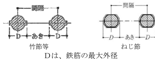
図 5.3.1 鉄筋相互のあき
