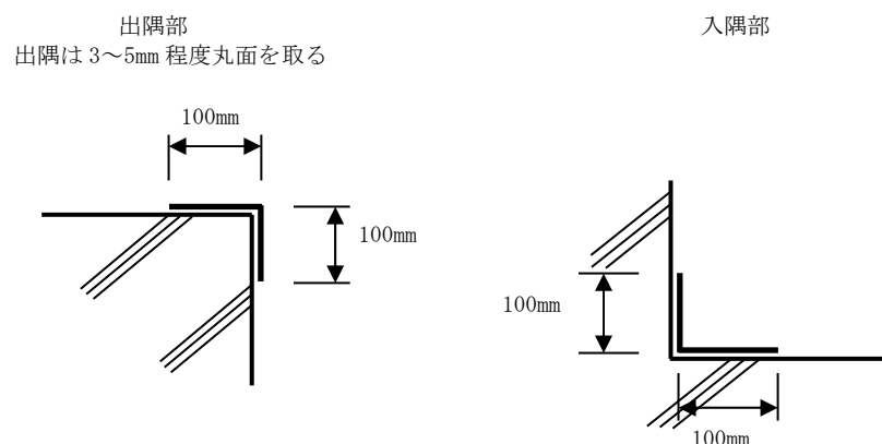
9.5.1 図 増し塗りの範囲
