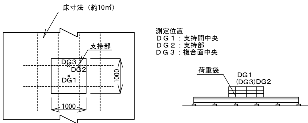
図—1 载荷試験方法
