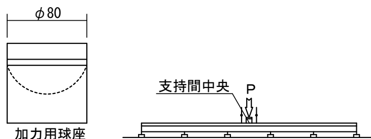
図一 2 局部曲げ試験方法
