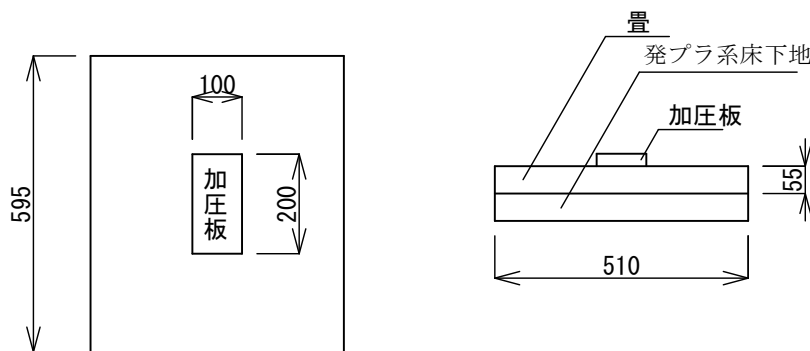
図—6 圧縮強度試験方法
