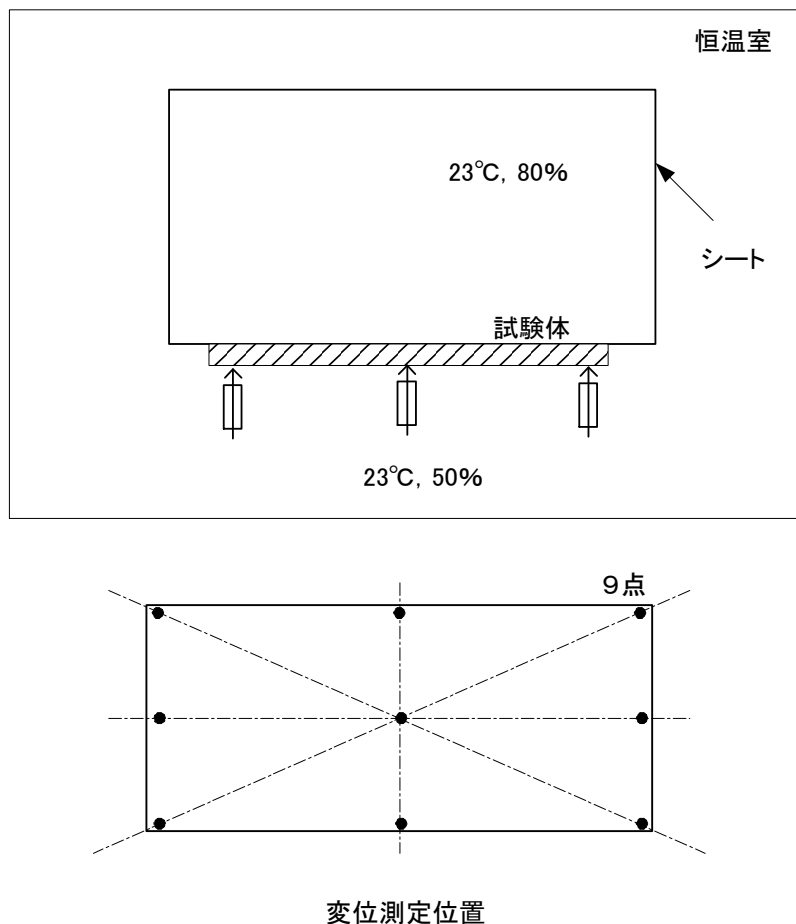
図－2 湿度変形試験方法の概要
