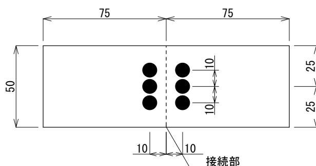
図一2 基板接続部 単位 (mm)
