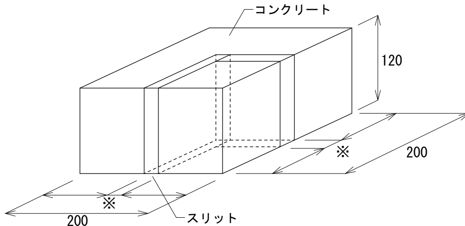
図－1 試験体概要図（単位 mm）
