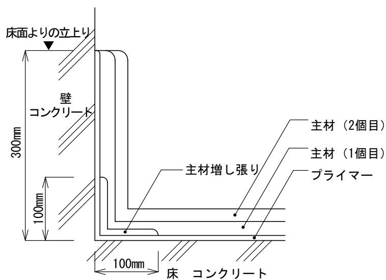
図－１ ポリマーセメント系塗膜防水材の構成
