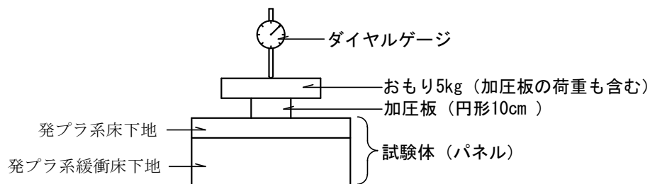
図一 5 静荷重圧縮試験方法
