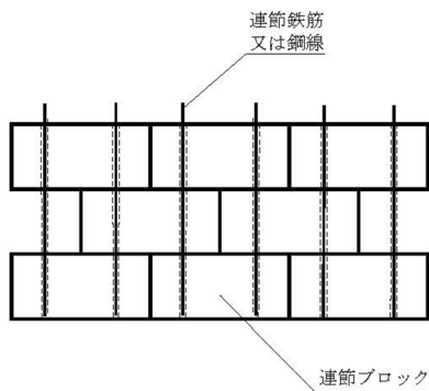
正面図
