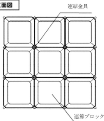
正面図
