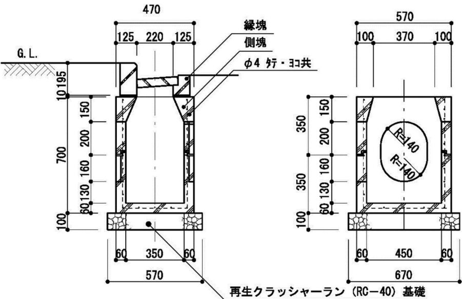
断面図
