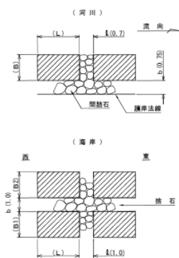
配置図
