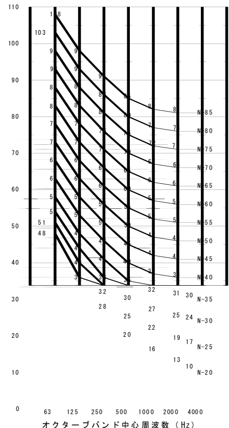
図1 建物の内部騒音に関する騒音等級の基準周波数特性(N曲線)
