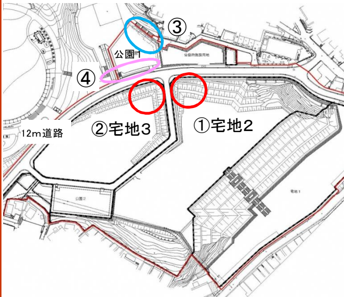
①②基礎杭の打ち込み ③地盤改良 ④12m道路と公園1の境になる擁壁の施工
