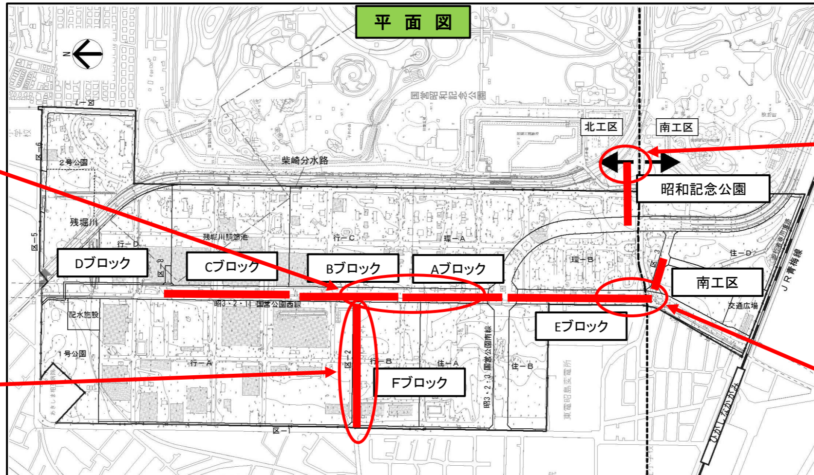
現場打マンホール工施工状況
