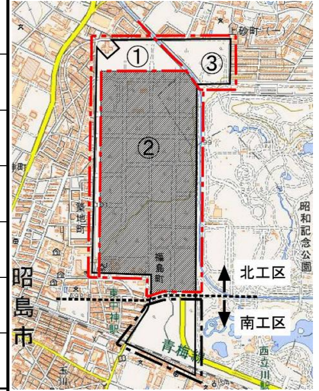
雨水本管工(ボックスカルバート)
