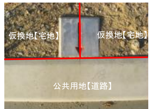
画地境界杭（コンクリート製） 90×90×600mm
