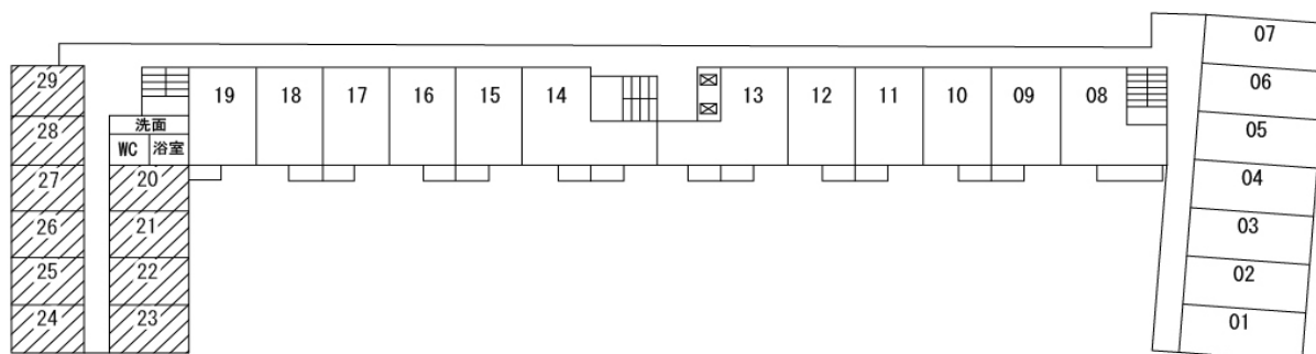
3階～5階平面図
