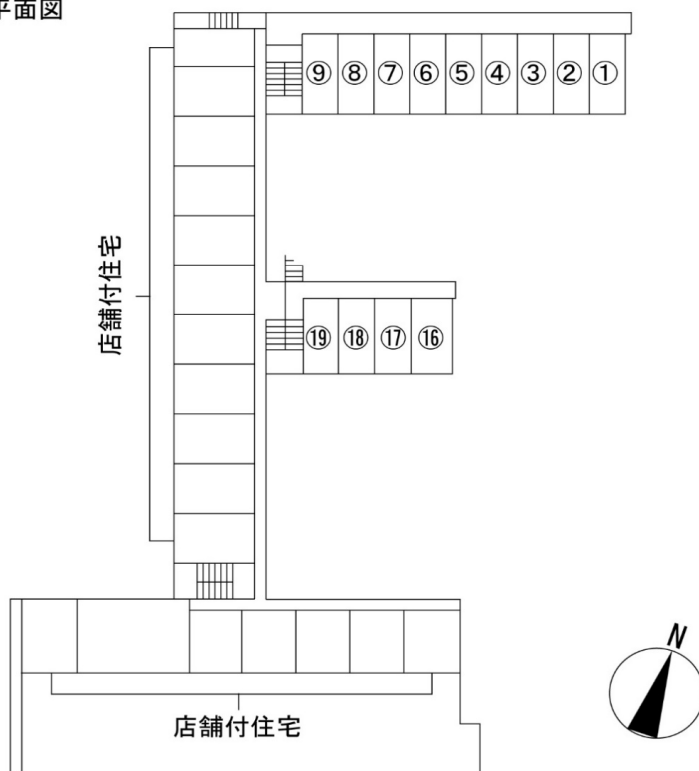
1号棟 2階平面図
