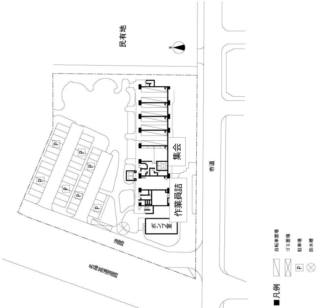
R西宮高畑町 配置図
