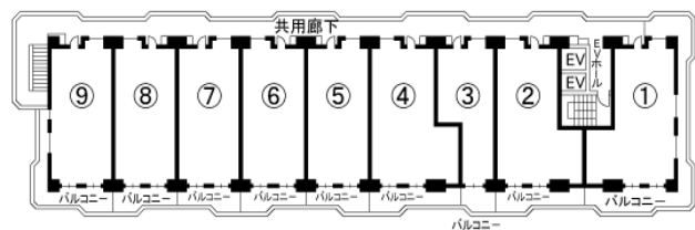
▲5階平面図
