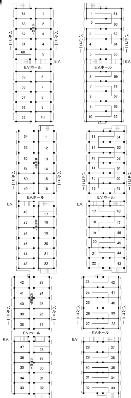
▲2・4・6・8・10・12・14階平面図
