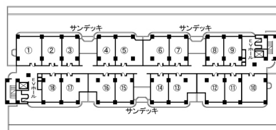
▲3階平面図
