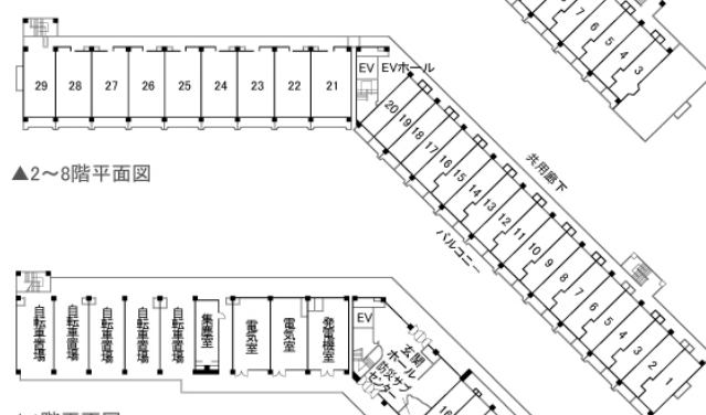
▲1階平面図
