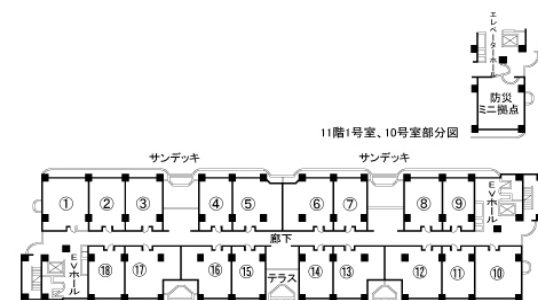
▲7・11・15・19・23階平面図
