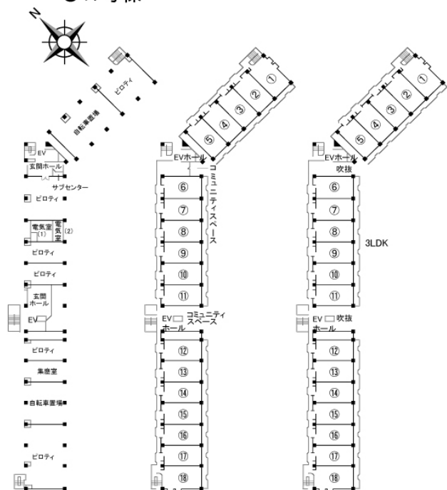
▲1階平面図 2・4・6・8・10・12階平面図
