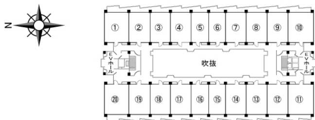
▲2～15階平面図 ※エレベーターは各階に停止します。
