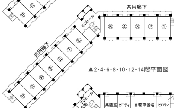
▲3・5・7・9・11・13・15階平面図
