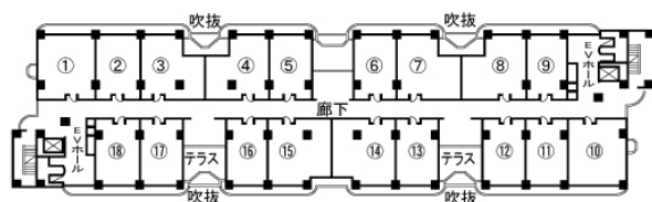
▲4・8・12・16・20・24階平面図
