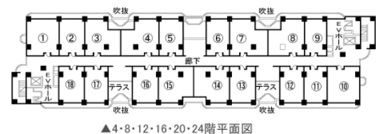
▲4・8・12・16・20・24階平面図
