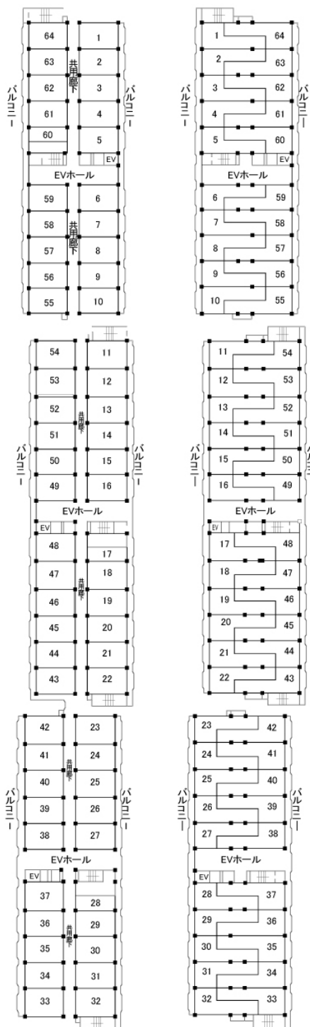
▲2・4・6・8・10・12・14階平面図 ▲3・5・7・9・11・13・15階平面図 ※エレベーターは2基1・2・4・6・8・10・12・14階に停止します。
