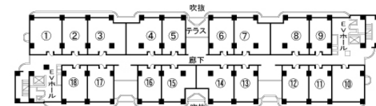
▲6・10・14・18・22階平面図
