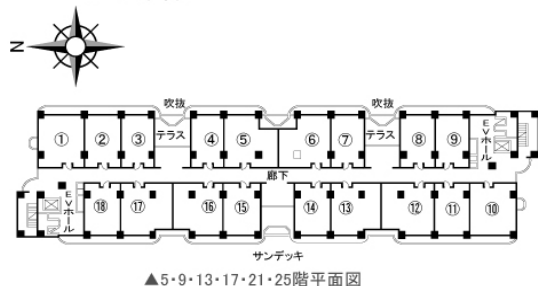
▲5・9・13・17・21・25階平面図
