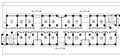
▲3階平面図
