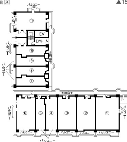
▲2～6階平面図
