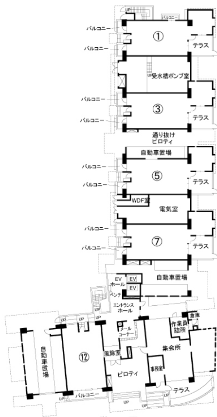
▲1階平面図
