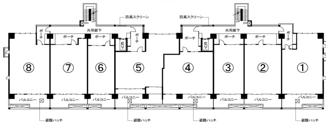
▲5階平面図
