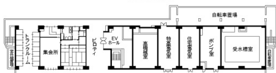
▲1階平面図
