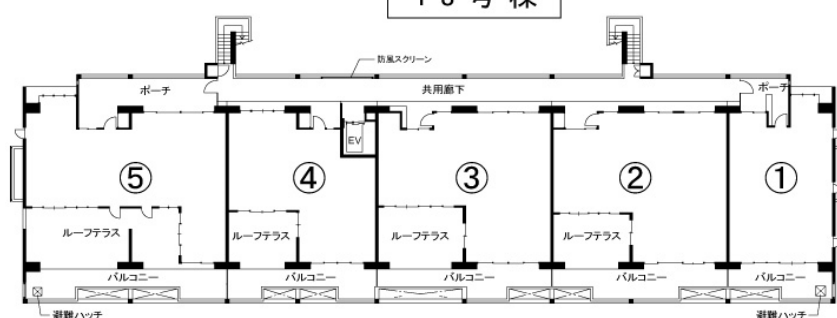
▲10階平面図
