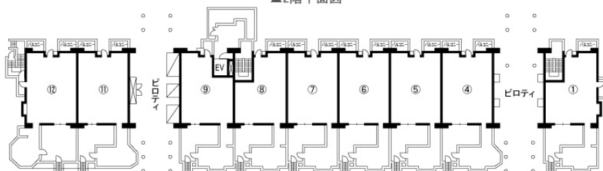
▲1階平面図
