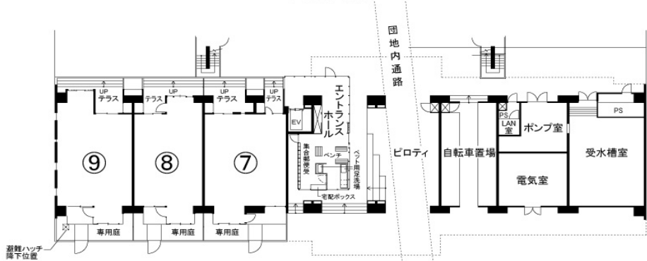
▲1階平面図
