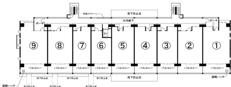
▲2階平面図
