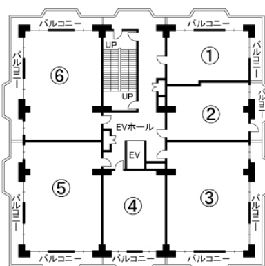
▲6～14階平面図
