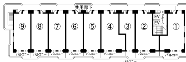
▲5階平面図
