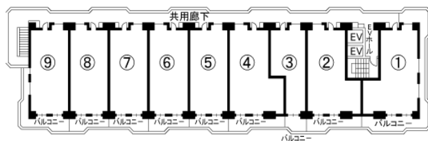
▲2～4階平面図
