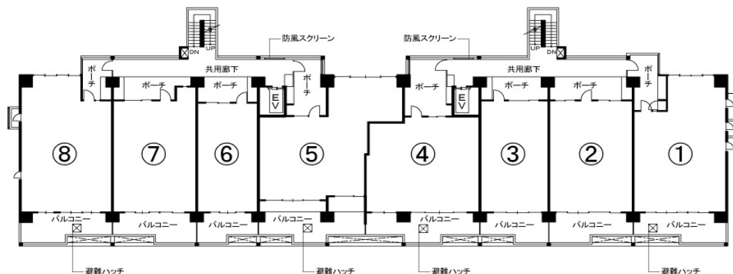
▲6階平面図
