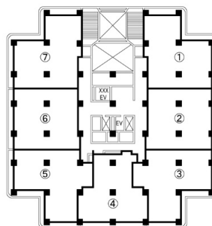
▲26～30階平面図
