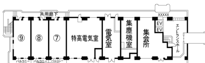
▲1階平面図
