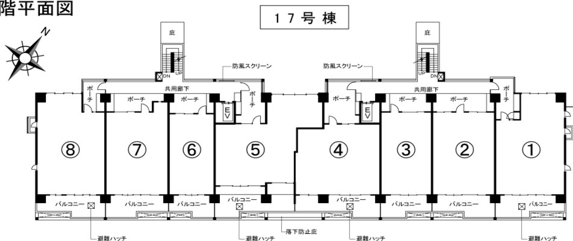
▲3階平面図
