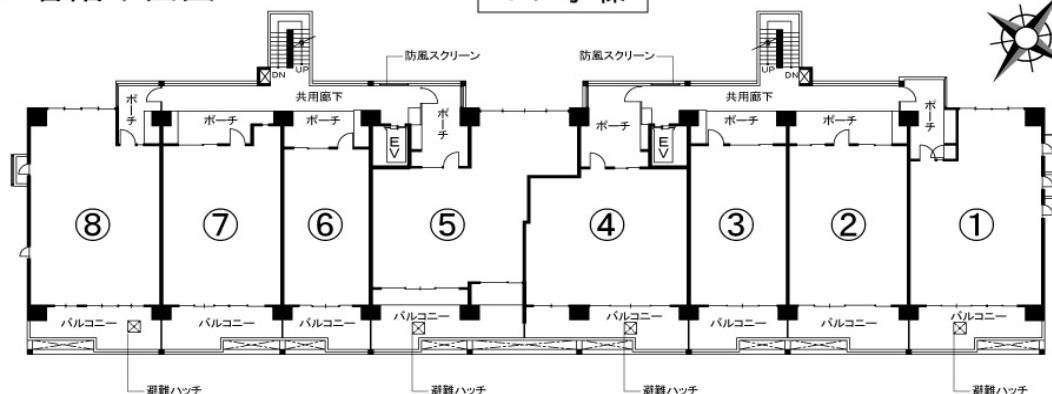
▲7階平面図
