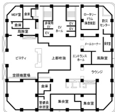
▲1階平面図
