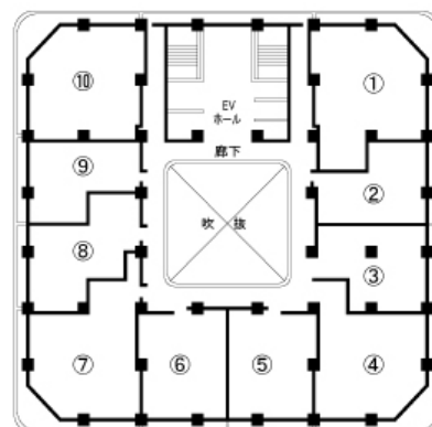
▲2～31階平面図
