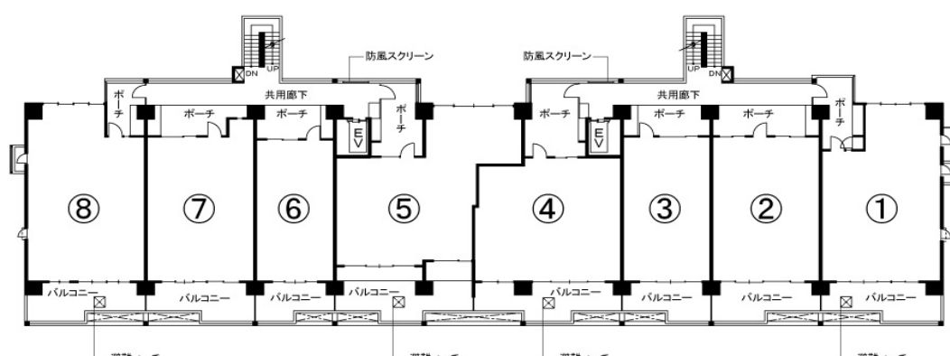
▲4階平面図
