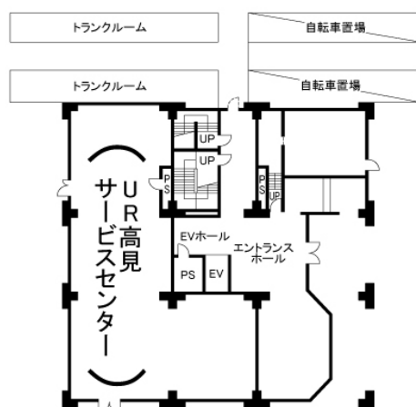
▲1階平面図
