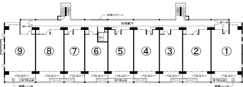
▲3階平面図
