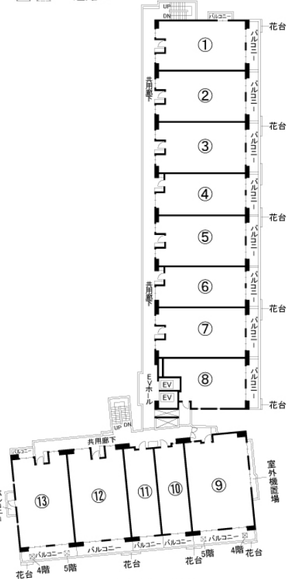
▲4・5階平面図
