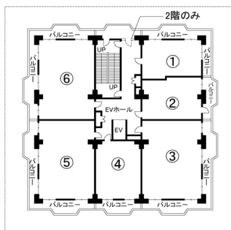
▲2～5階平面図
