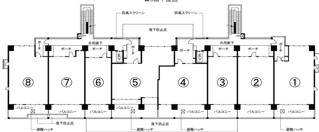
▲2階平面図
