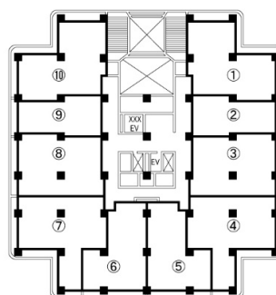
▲19～25階平面図
