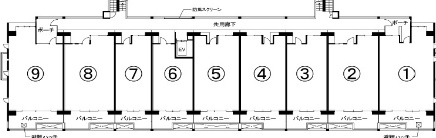
▲5階平面図
