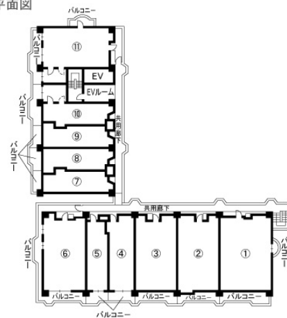
▲7～13階平面図
