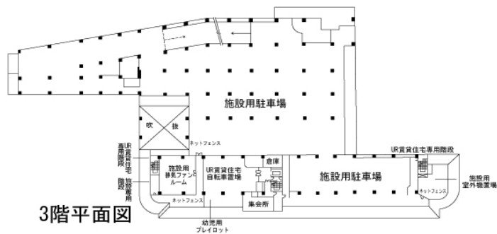
4階平面図
