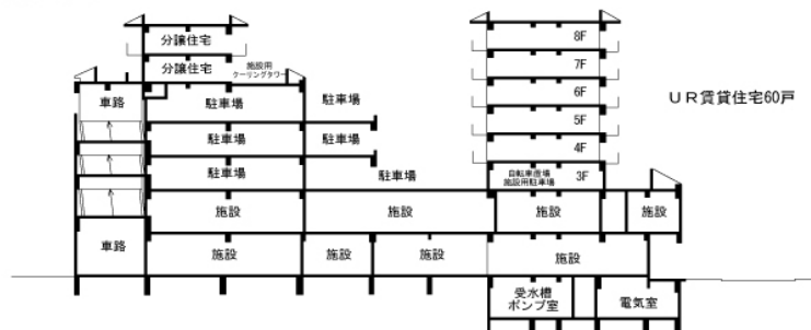
断面図
