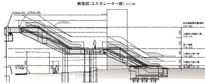
【計画断面図(ESC部)】
