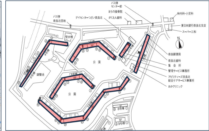
配置図
