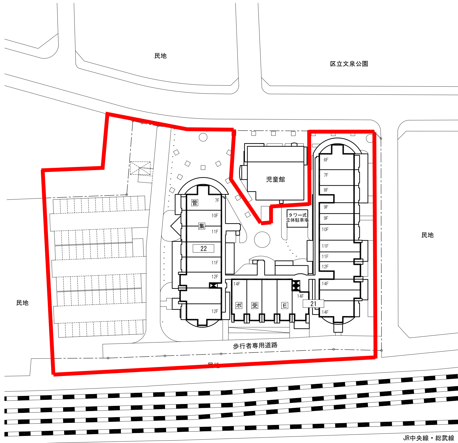
アーバンライフ亀戸 配置図
