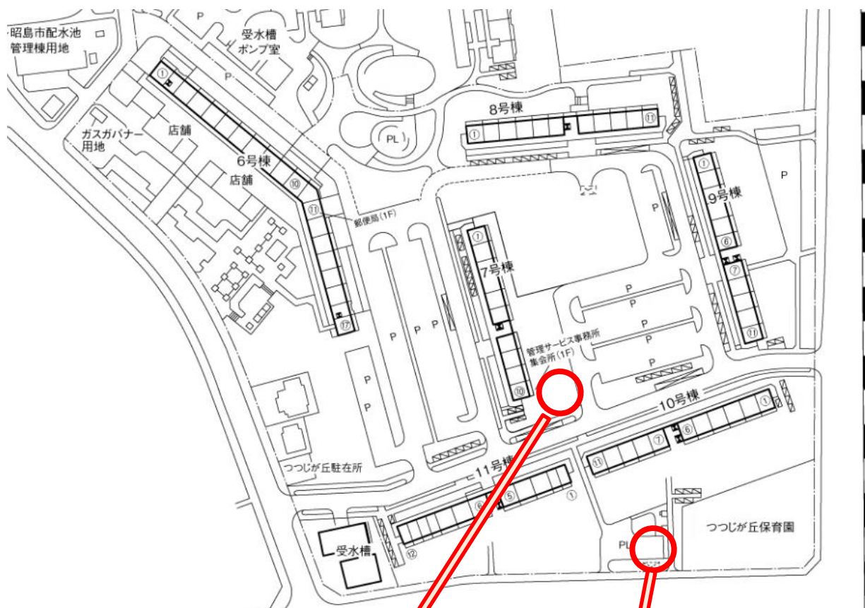
昭島つつじが丘ハイツ 配置図
