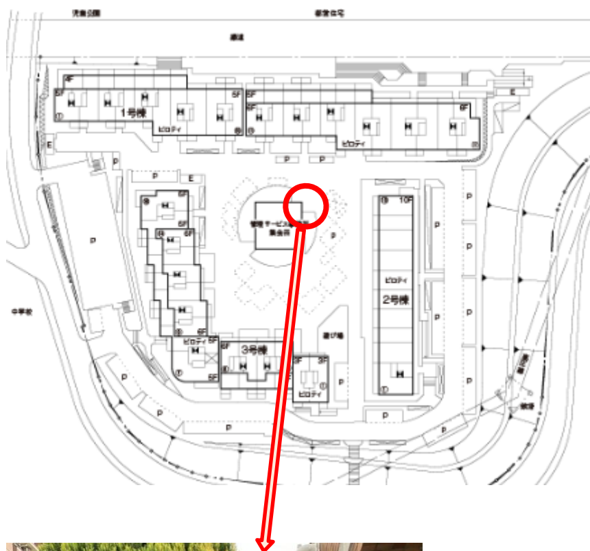
多摩 NT ベルコリーヌ南大沢 配置図
