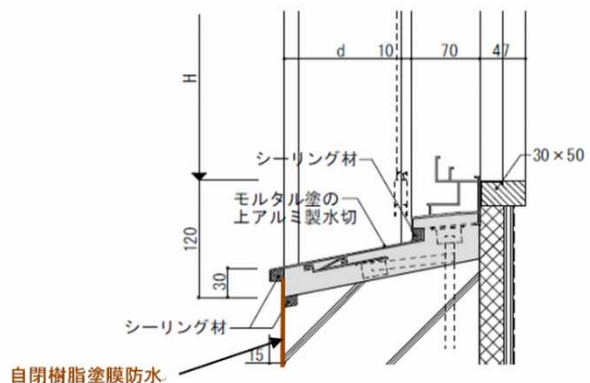
図2：開口部廻り塗布範囲参考図（断面）
