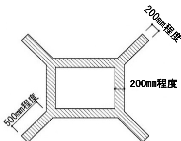
図3：開口部廻り塗布範囲参考図（立面）
