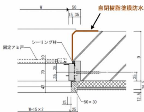
図1：開口部廻り塗布範囲参考図（平面）
