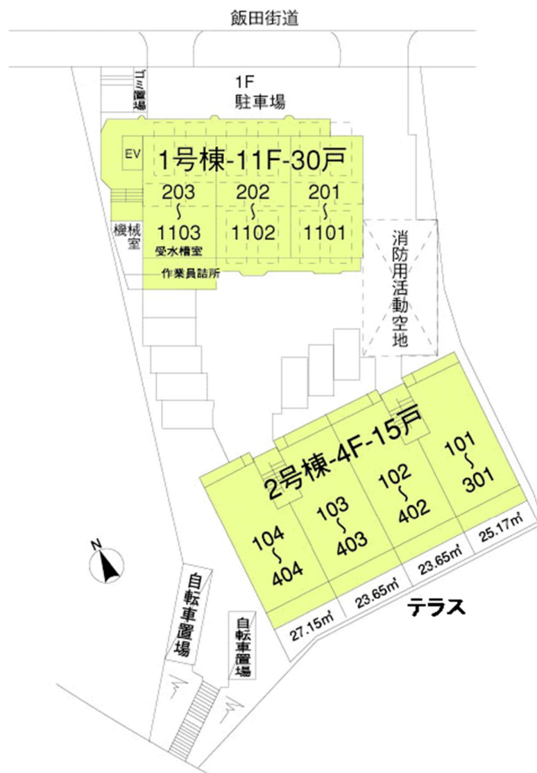
配置図
