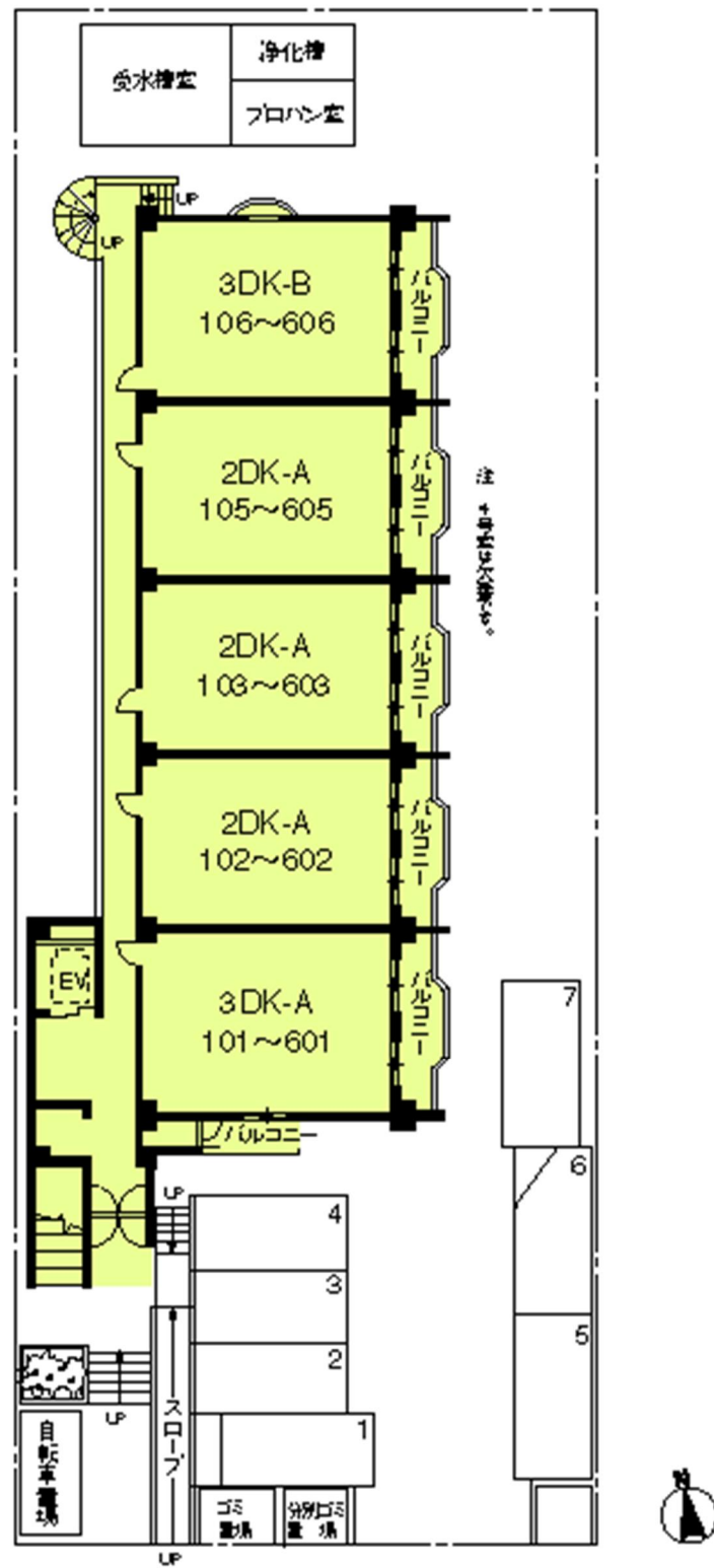
配置図
