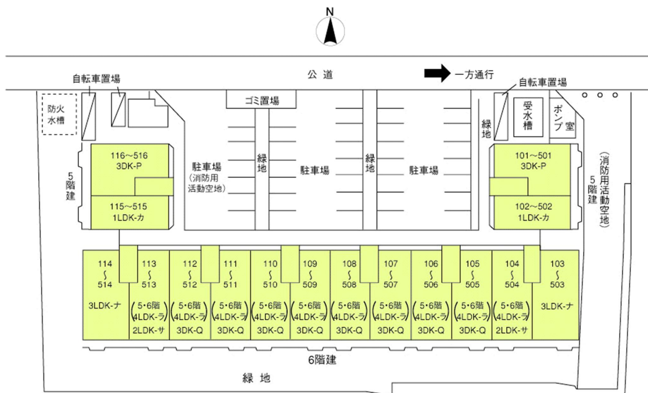
配置図
