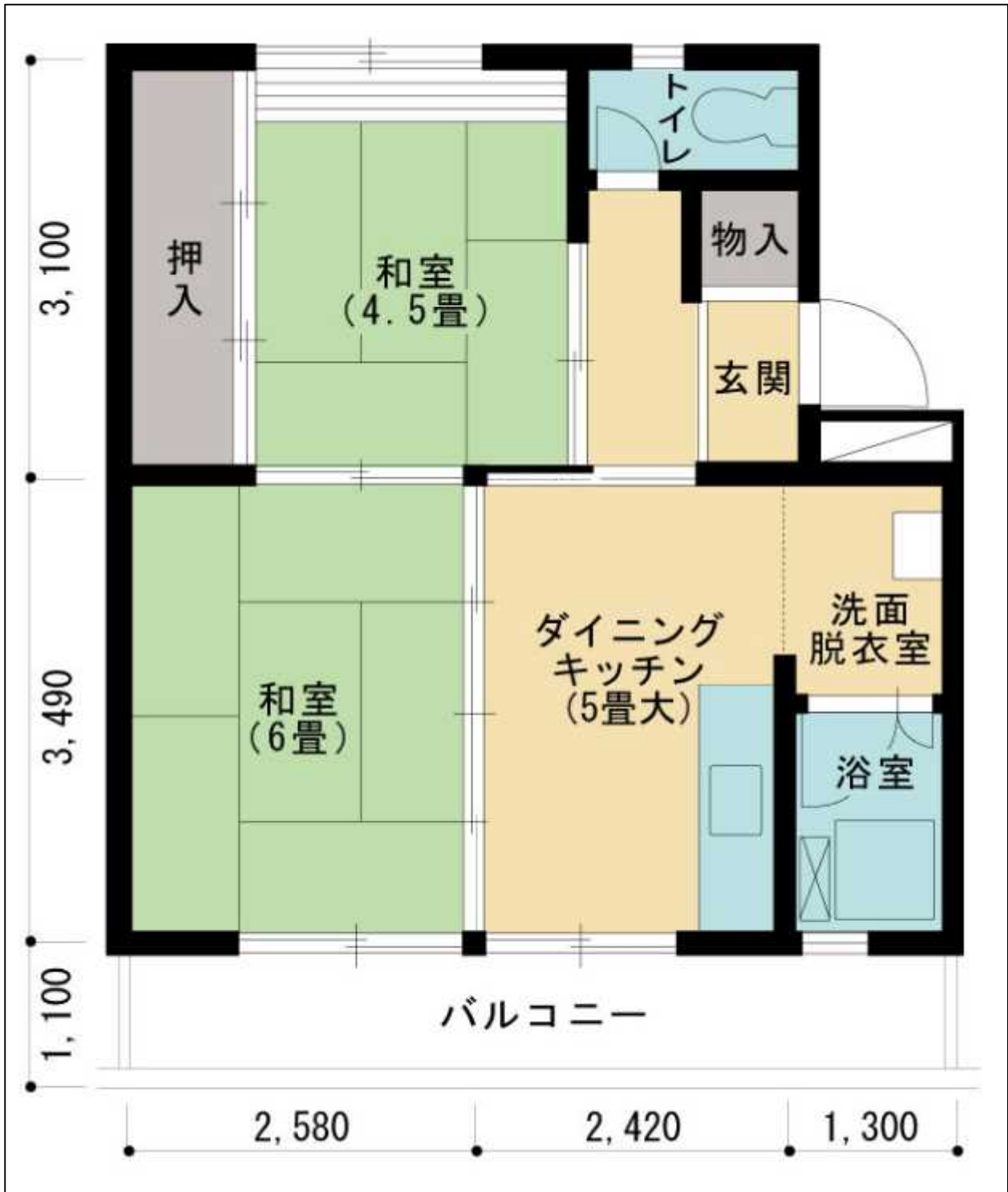
<募集住戸 間取図>30号棟 304号室(2DK/38.16㎡)
