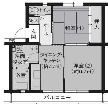
改良後の間取例
