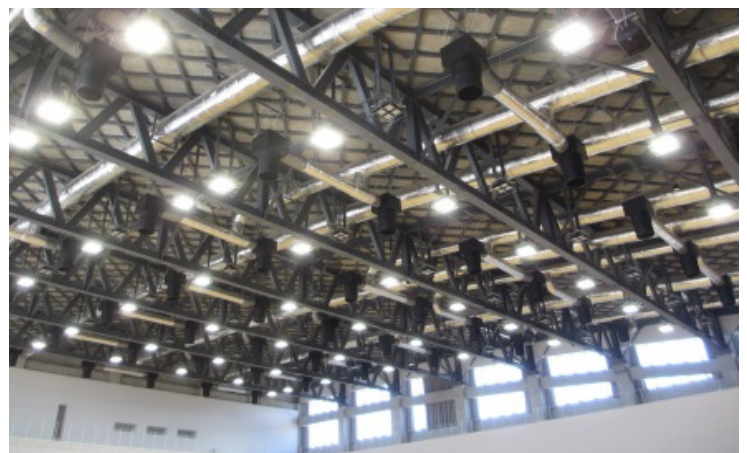
◆地震対策のため、吊天井を改修
