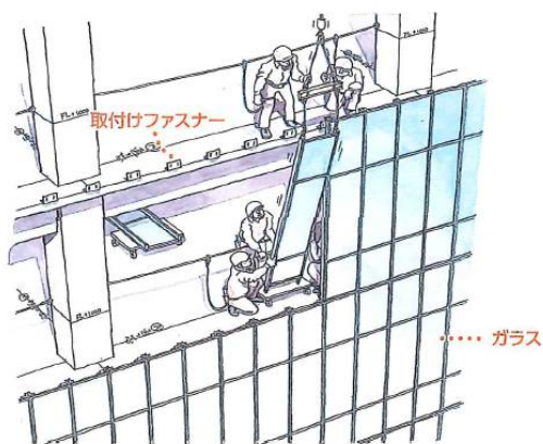
【出展】イラスト「建築施工改訂版」 （一般社団法人日本建設業連合会関西支部）
