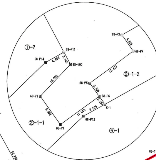
拡大図A S=1:500
