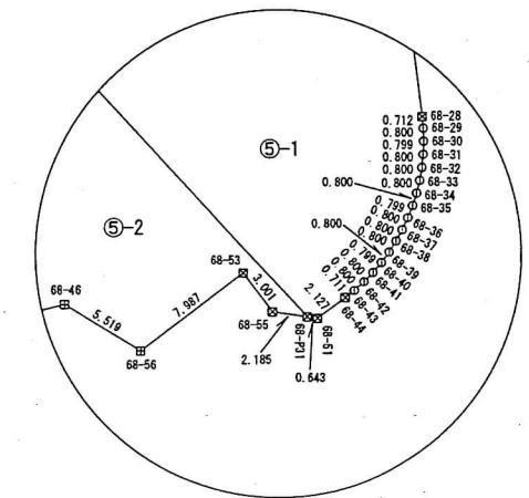
拡大図B S=1:500
