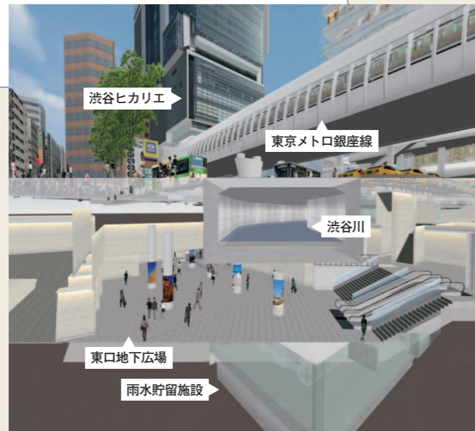
渋谷駅東口断面図イメージ
